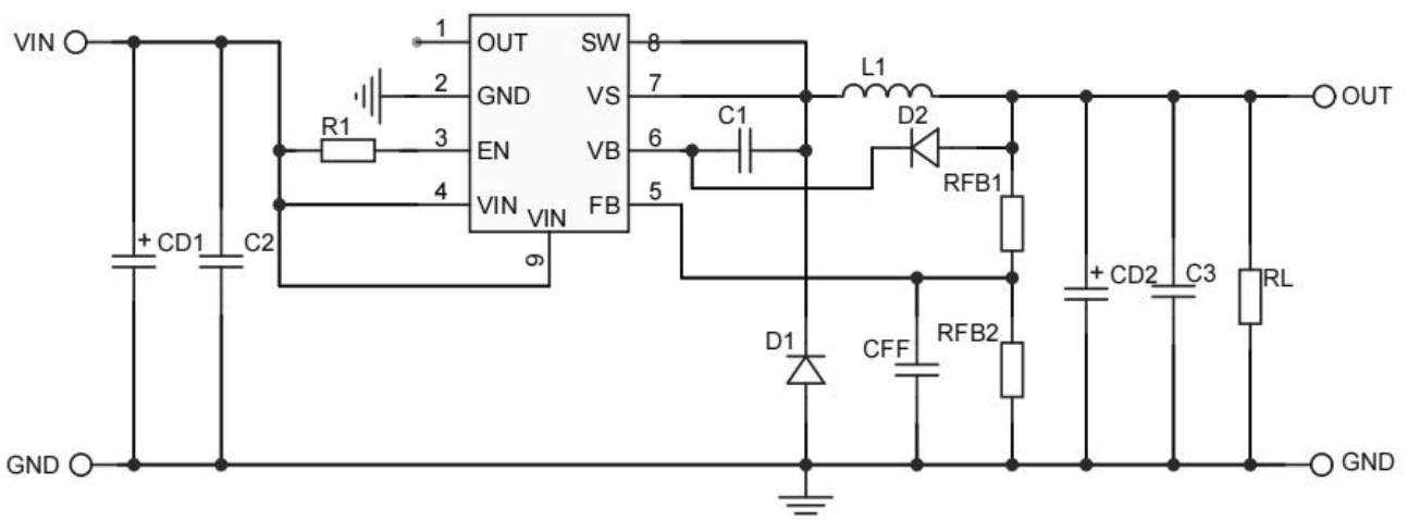
APP2: V_{OUT}=10\sim15V
